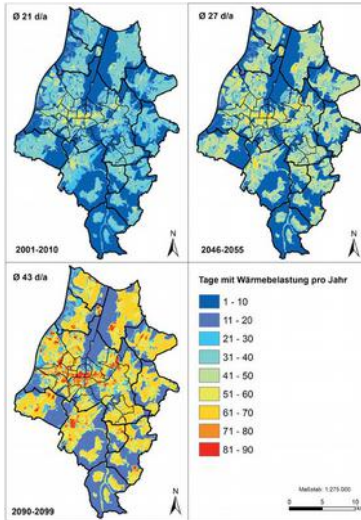
Durchschnittliche jährliche Anzahl der Tage mit Wärmebelastung (PMV) im Gebiet des NVK für die Dekaden 2001-2010, 2046-2055 und 2090-2099;
